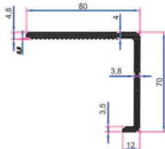
70x80 mm PERVAZ
