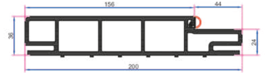
200mm KAPI KASA
