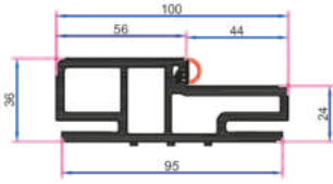
100mm KAPI KASA
