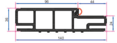
140mm KAPI KASA
